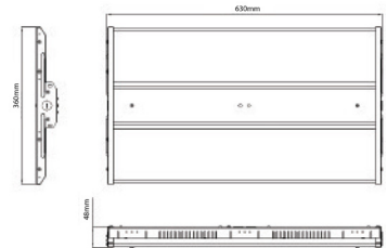
220W Dimensions
